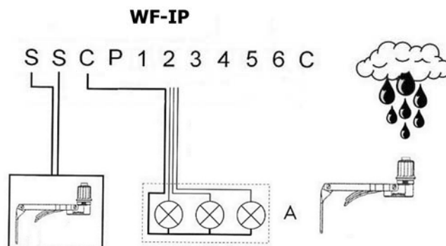
Čidlo srážek se zapojením "normálně uzavřeno" NC
